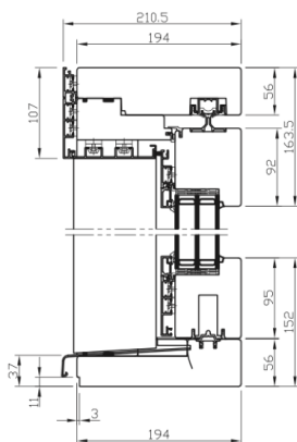
Pystyleikkaukset
