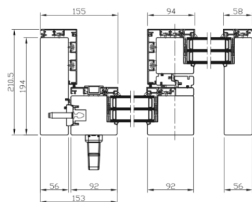
Vaakaleikkaus
